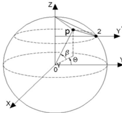
Figura 5. Ángulos para el sistema de coordenadas esférico
