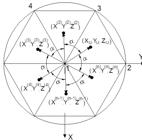
Figura 10. Transformación de rotación
