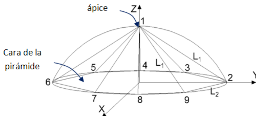
Figura 3. Pirámide dividida en 8 partes. n=8 , NCP=8
