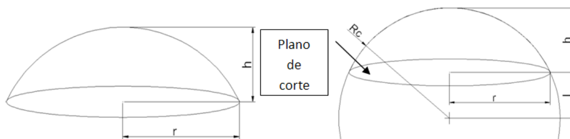
Figura 2. Sector esférico de una esfera
