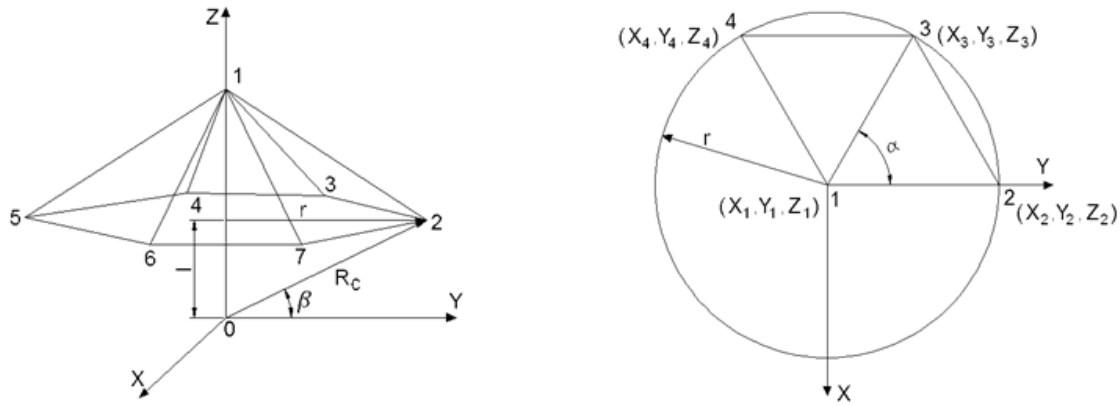
Figura 4. Pirámide y proyección de las dos primeras cara de la pirámide sobre el plano X-Y
