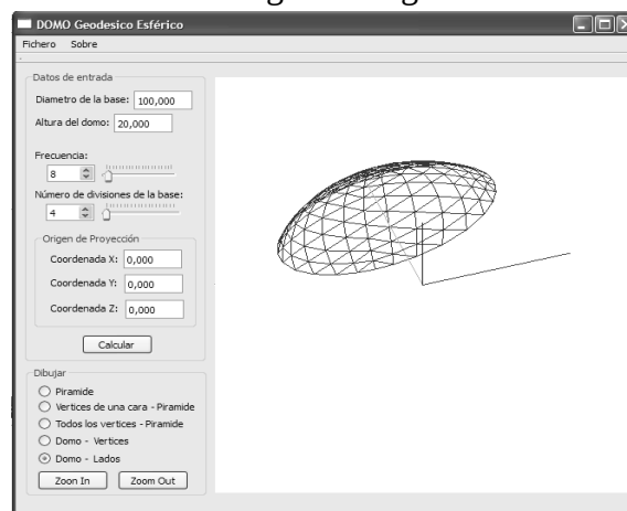
Figura 15. Ventana principal del software DOMO Geodésico Esférico
