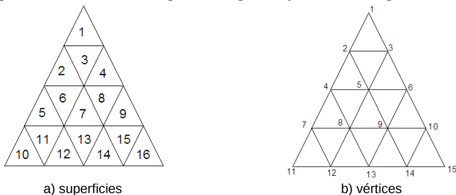
Figura 7. Número de subdivisiones de una cara de la pirámide con f=4 , NSCP=16 y NVCP=15
