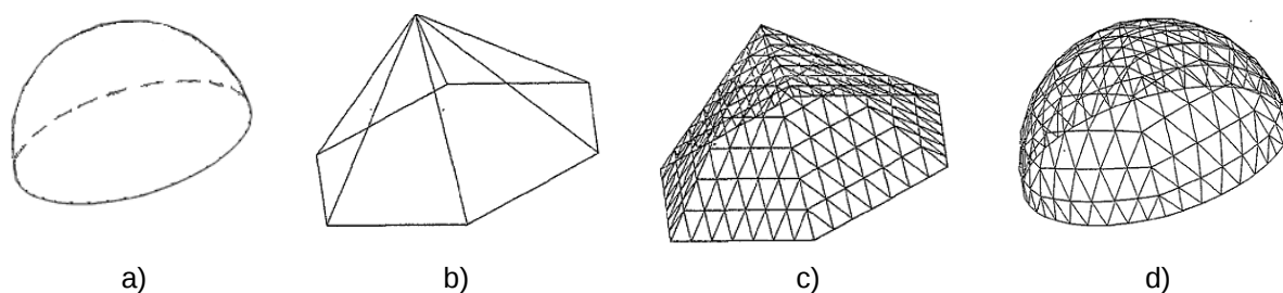
Figura 1. Etapas para la creación del modelo alámbrico de un domo geodésico esférico
